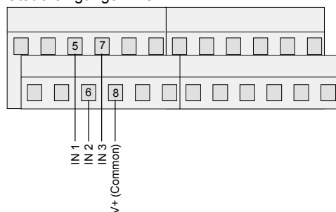
Steuereingänge ETC 24
