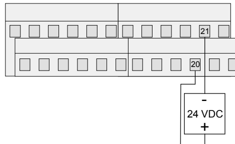
DC-Fremdspeisung ETC 12/14/24
